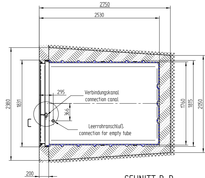
SCHNITT B-B
