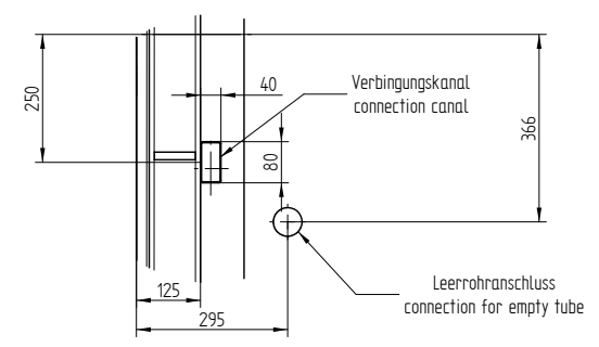
EINZELHEIT C
