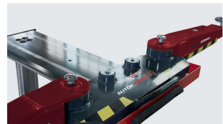
Verschiebbare Schwenkarmlastaufnahme
