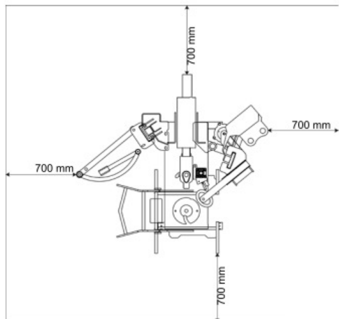
Abb. Aufstellfläche
