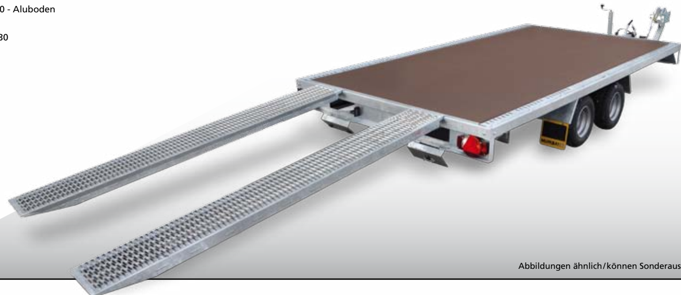
Seilwinde mit Seil und 3-fach tiefenverstellbarer Halterung, serienmäßig verbaut
