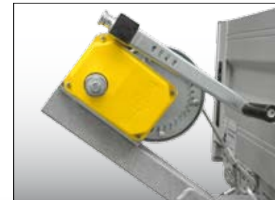
Seilwinde mit Seil und 3-fach tiefenverstellbarer Halterung, serienmäßig verbaut
